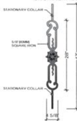
HFBX.F
